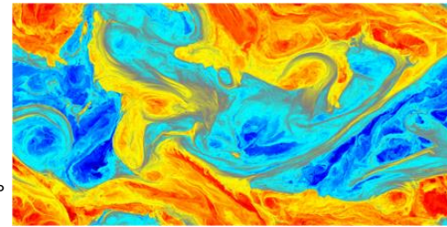
富岳によるシミュレーションで得られた降着円盤の磁場揺動分布
